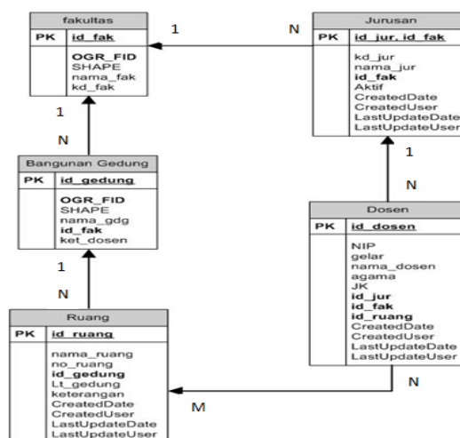
Gambar 2 Diagram Keterhubungan Antar tabel pada Sistem
