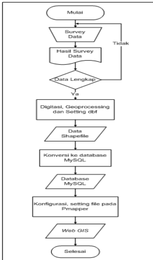
GAMBAR 1 Diagram Alir Proses Pembuatan WEB-GIS
